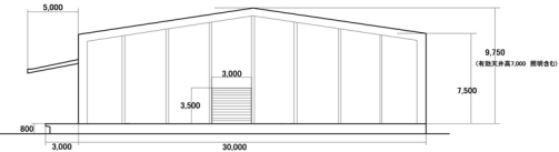
断面图
