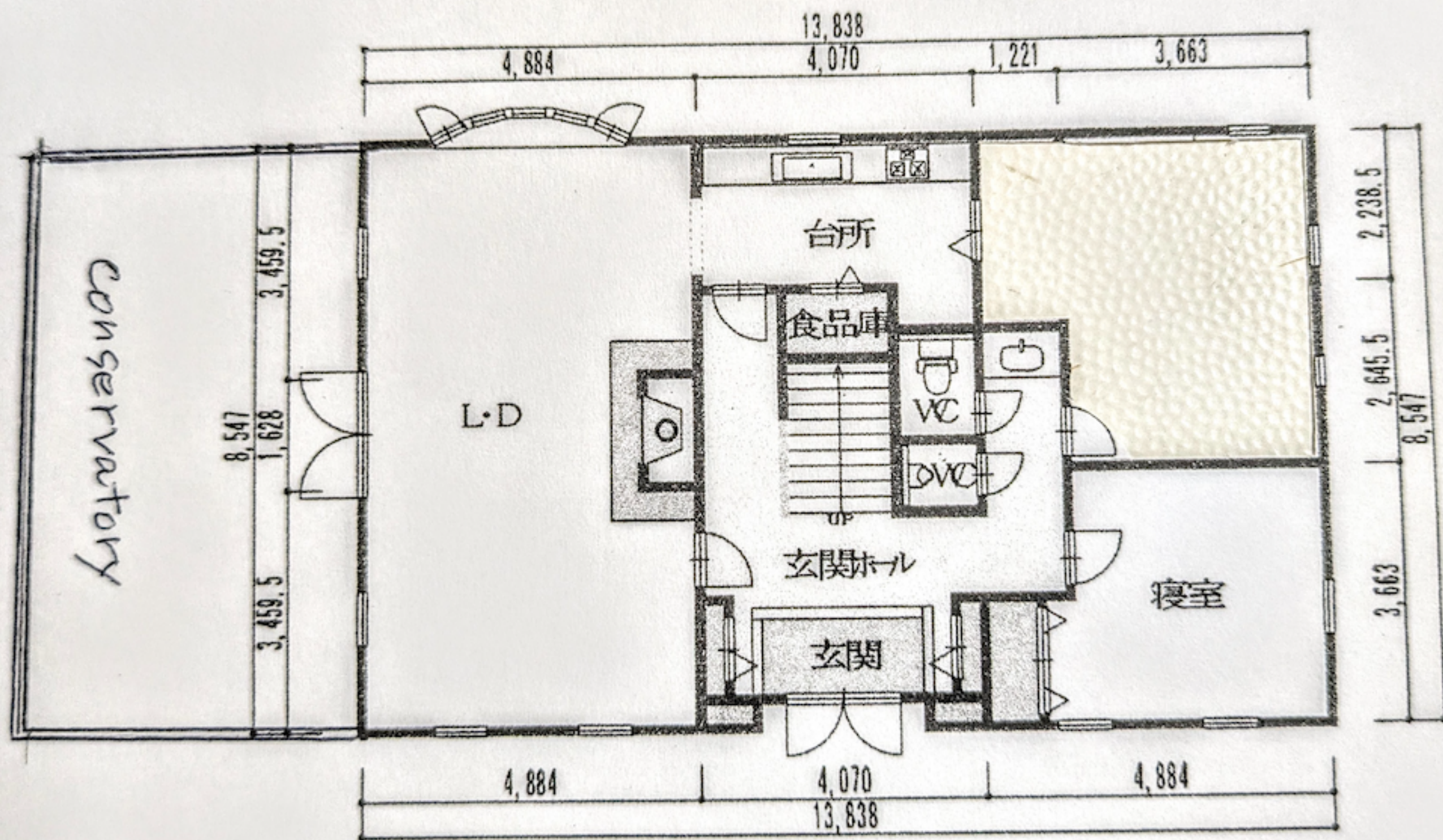
一階平面 116.62m 2 (35.34坪)
