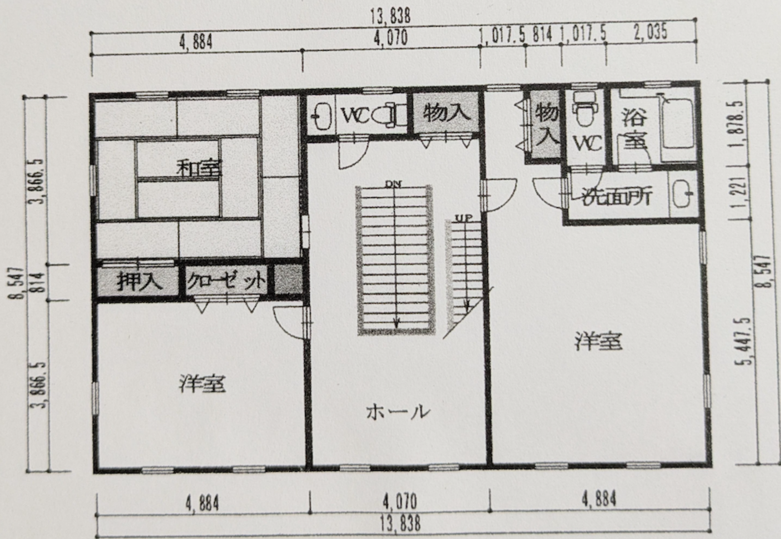
二階平面 118.27m 2 (35.84坪)
