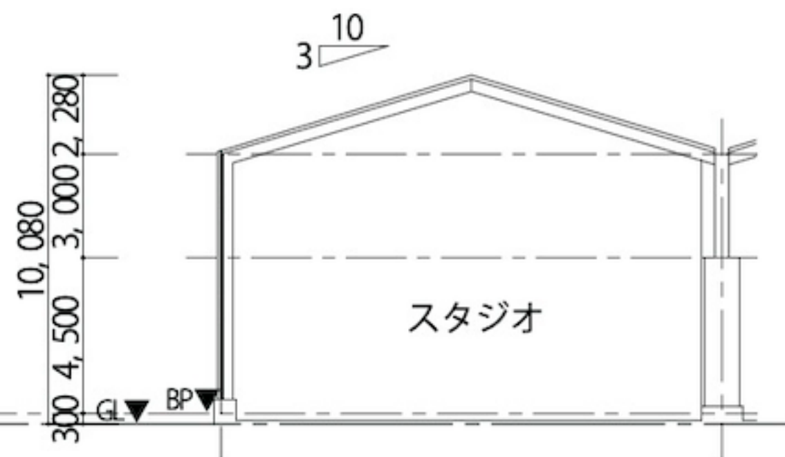
C-C断面
