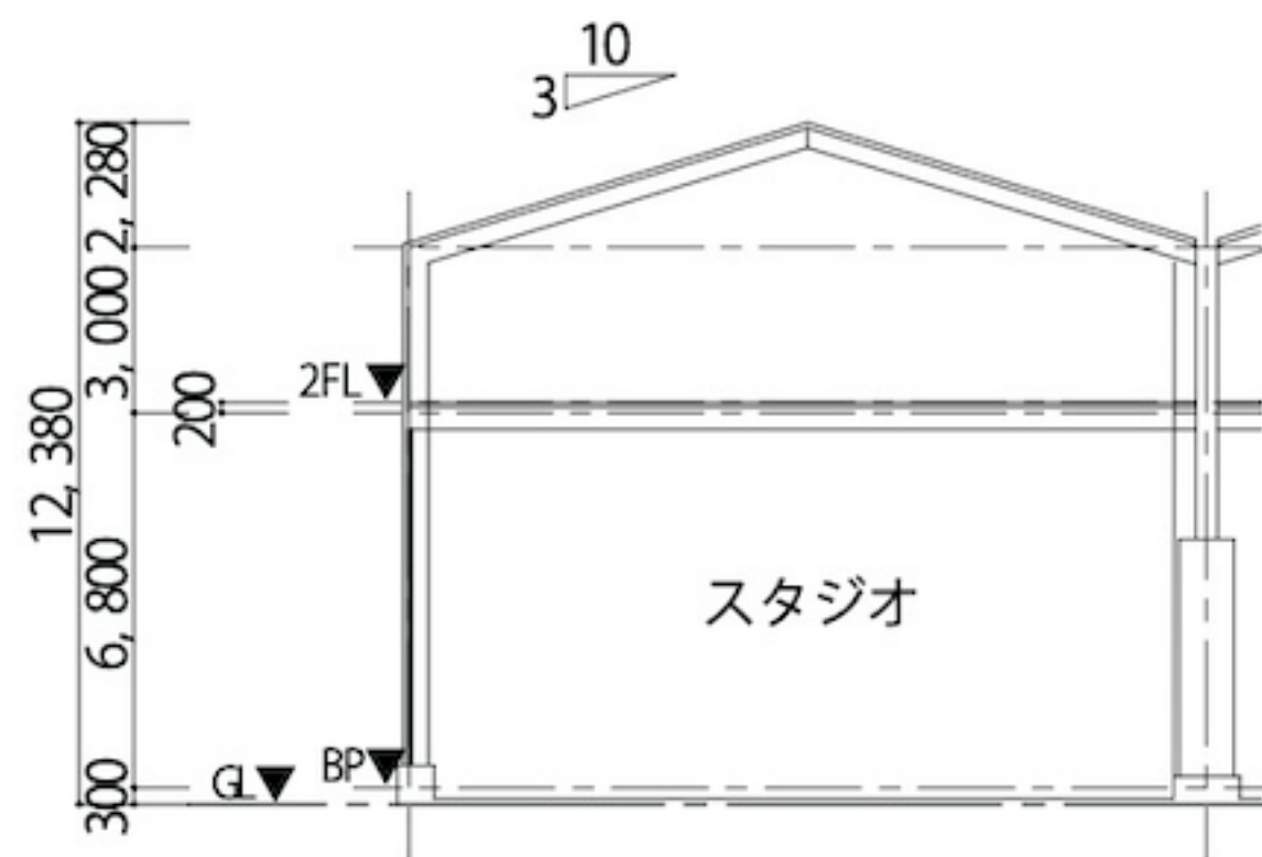
B-B断面
