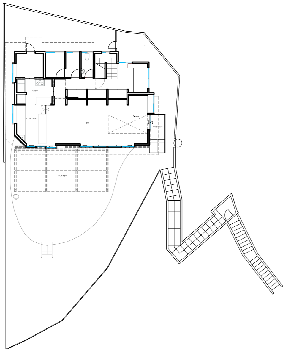
配置図 S=1/200
